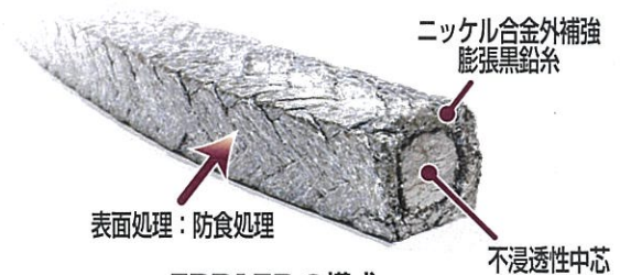
EDP15Pの構成
